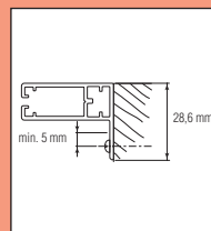
Standard sido-kanal, kort
