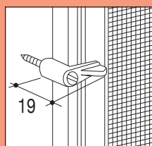
Vridbeslag bygger 9 mm
