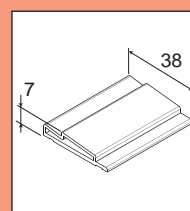
Bottenlist, 6,5° vinkel
