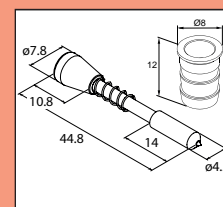
Fjäderstift + metall bussning, som sätts i det borrade hålet.
