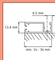
Sidokanal
