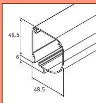
kassett profil
