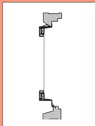
Träram med aluminium
