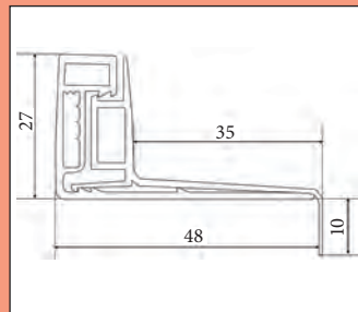
Djup 43 mm
