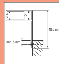
Sidokanal, lång
