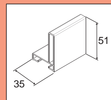
Monteringsprofil
