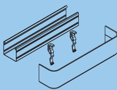
Fusion utanför nisch Frontprofil är färdigmått +22 mm
