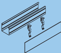
Fusion i nisch Frontprofilen är färdigmått +8 mm
