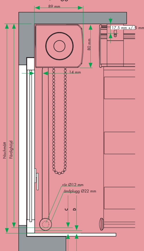
Tak/vägg – kassett
