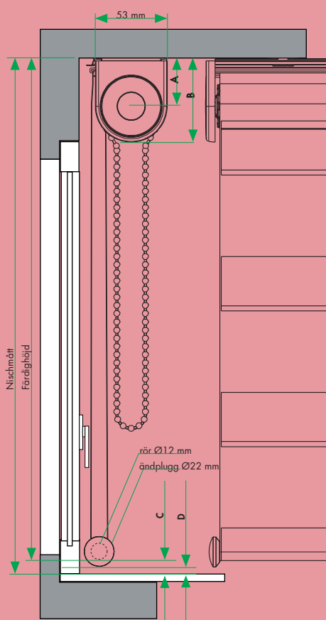
Tak/vägg – kassett
