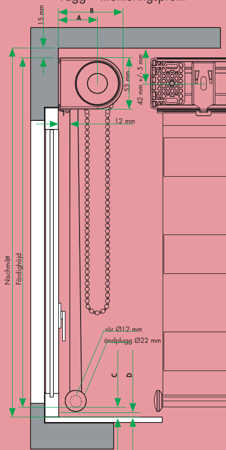
Vägg – monteringsprofil
